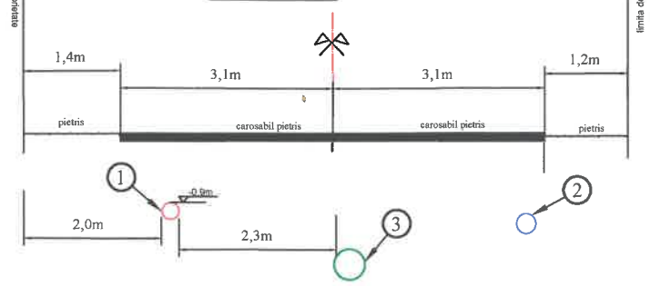
Strada SPIRU HARET DS Sectione transversala 2-2 Scara 1:100
