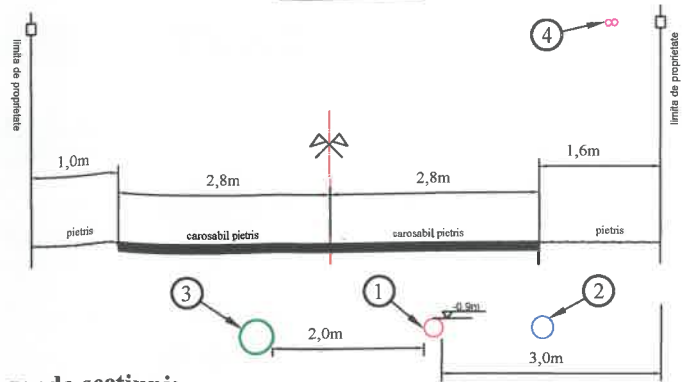
Strada SPIRU HARET Sectione transversala 1-1 Scara 1:100
